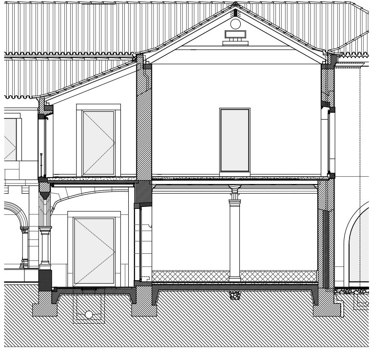
Sezione di dettaglio 03 - Chiostro ala nord
