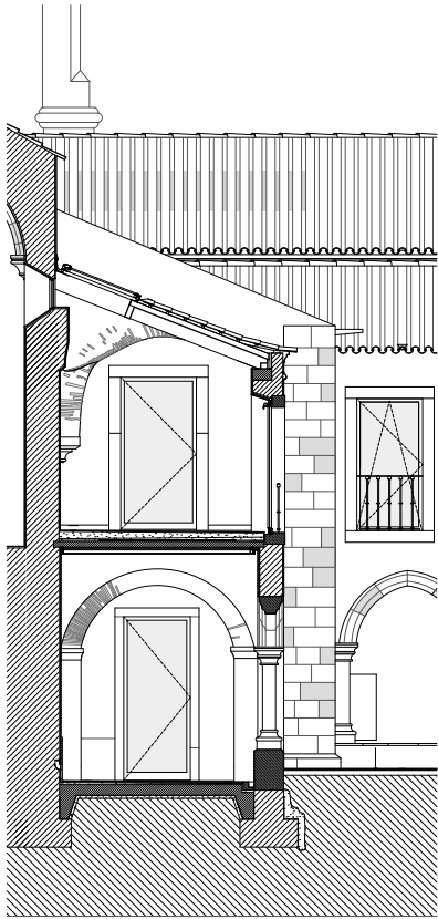
Sezione di dettaglio 02 - Chiostro ala sud
